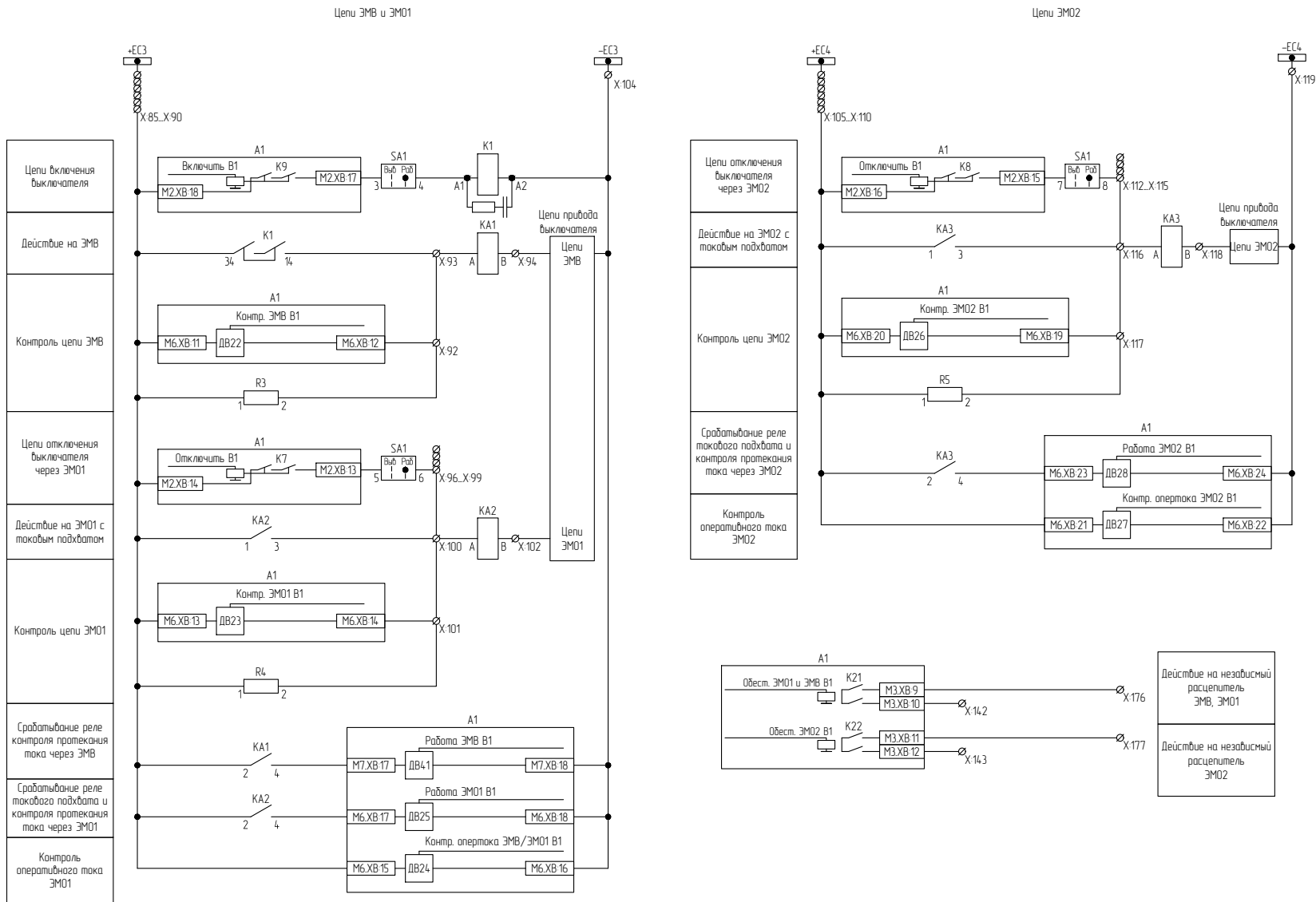
Рисунок В.3 – Схема электрическая принципиальная (часть 3)
